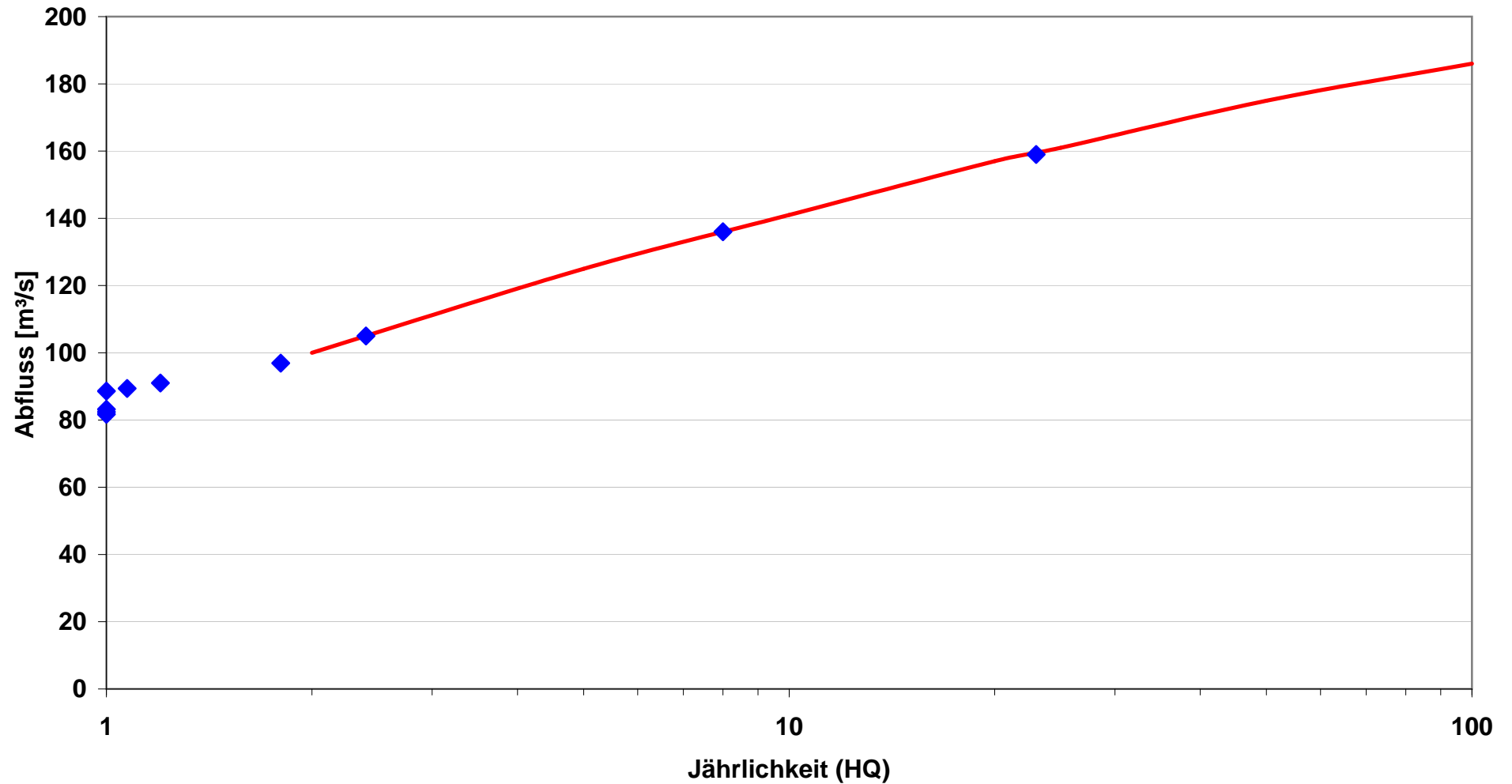
Diagramm der Verteilungsfunktion Friedrichsthal
