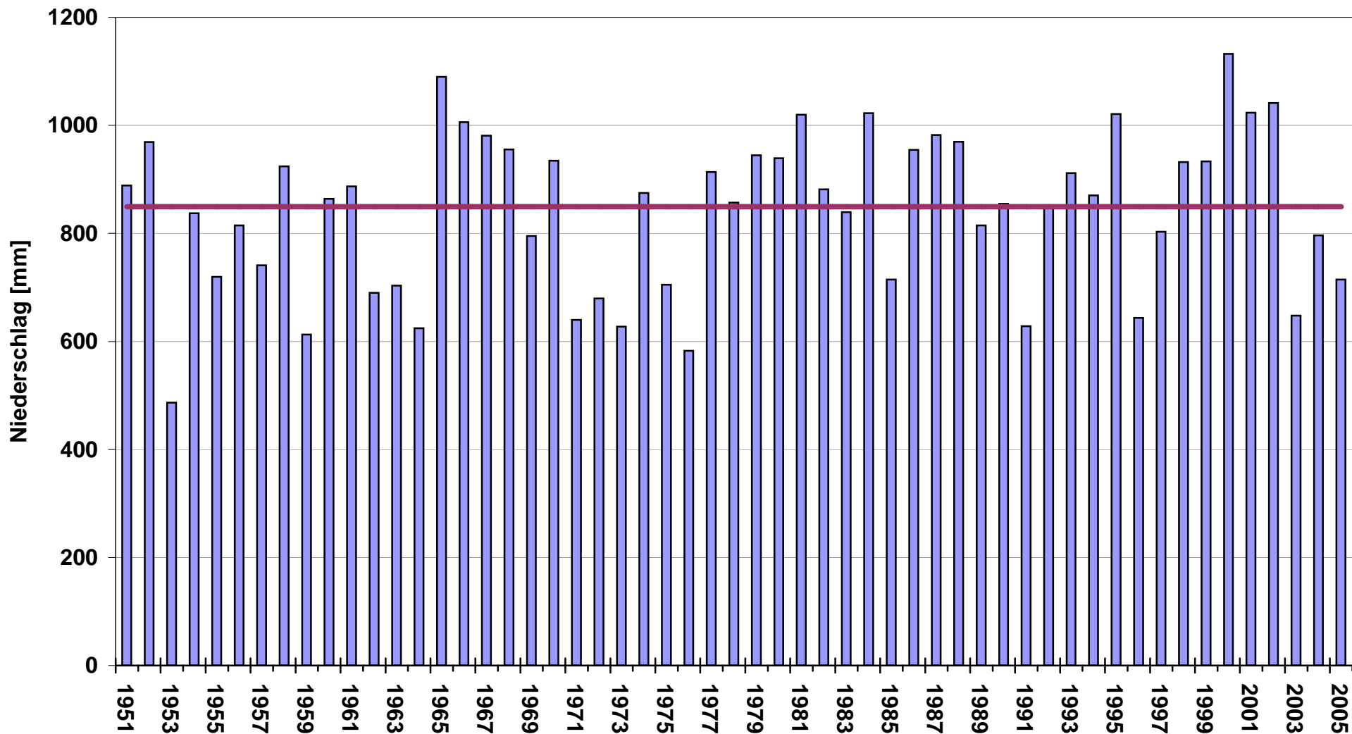
Pegel Martinstein Jährliche Niederschlagshöhen 1951 bis 2005 im Vergleich zur mittleren jährlichen Niederschlagshöhe der Normalperiode 1961-1990
