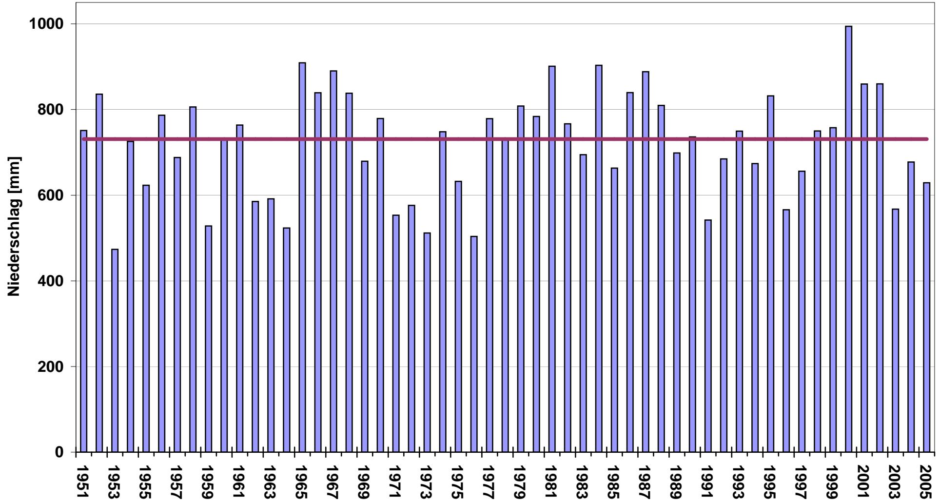
Pegel Kellenbach Jährliche Niederschlagshöhen 1951 bis 2005 im Vergleich zur mittl. jährl. Niederschlagshöhe der Nomalperiode 1961 -1990
